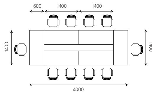
회의용 테이블 (A TYPE) W4000XD1400XH750
